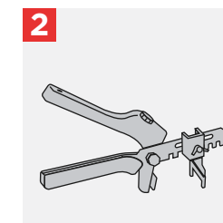
Pinza de presión
